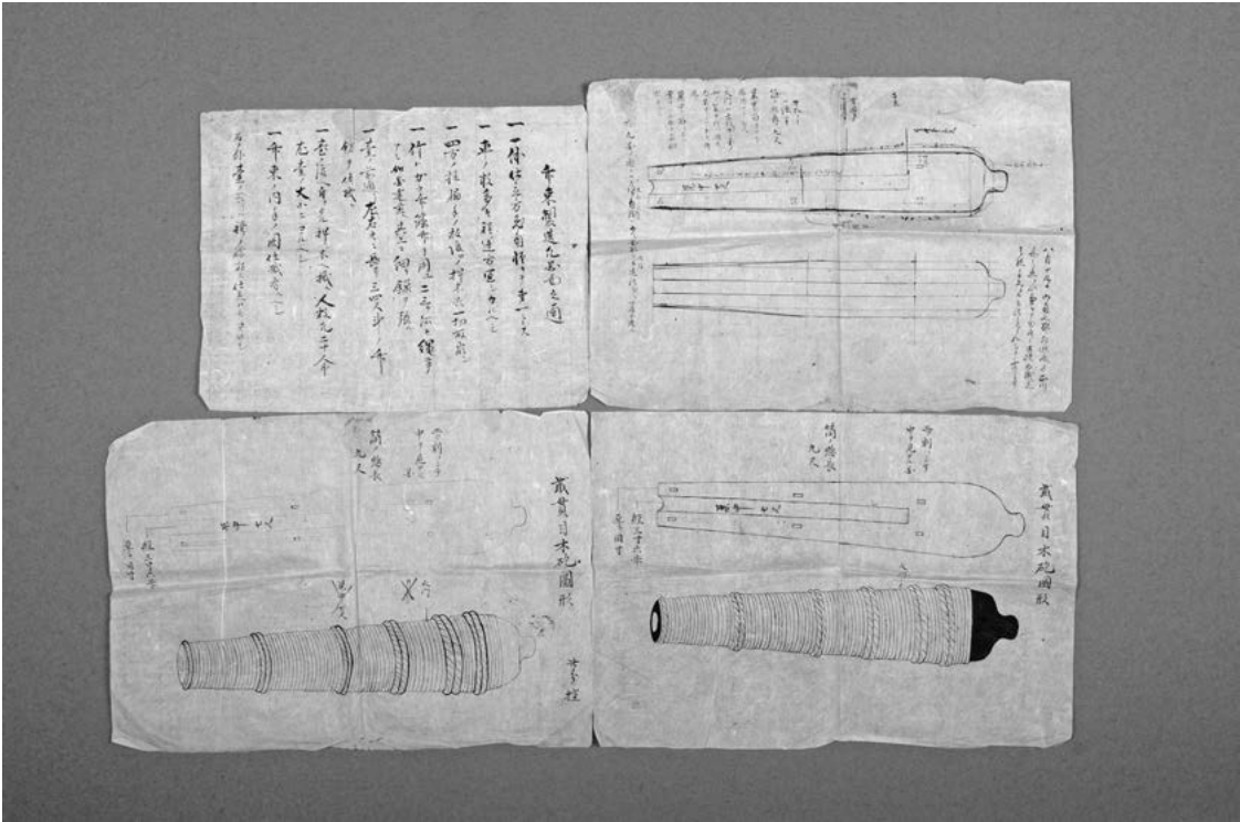
9～10 式貫目木砲図形 / 13 竹束製造凡図面之通（今村家文書）
